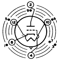
INDEX=LARGE LUG ● = PIN CUT OFF
